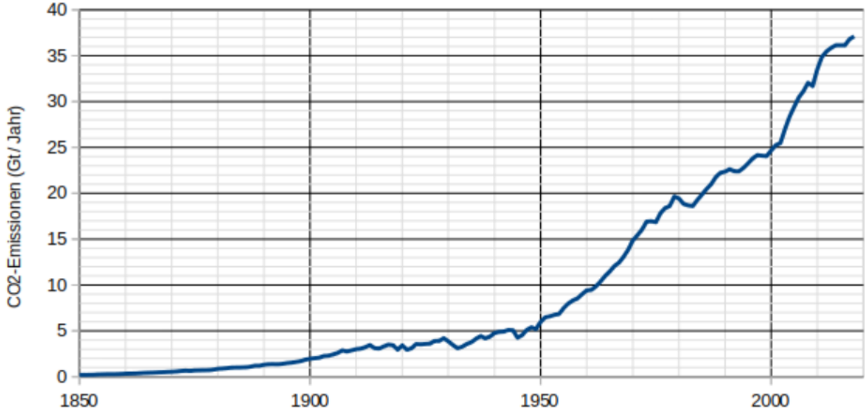
— Jährliche CO2-Emissionen (Gt/Jahr)
